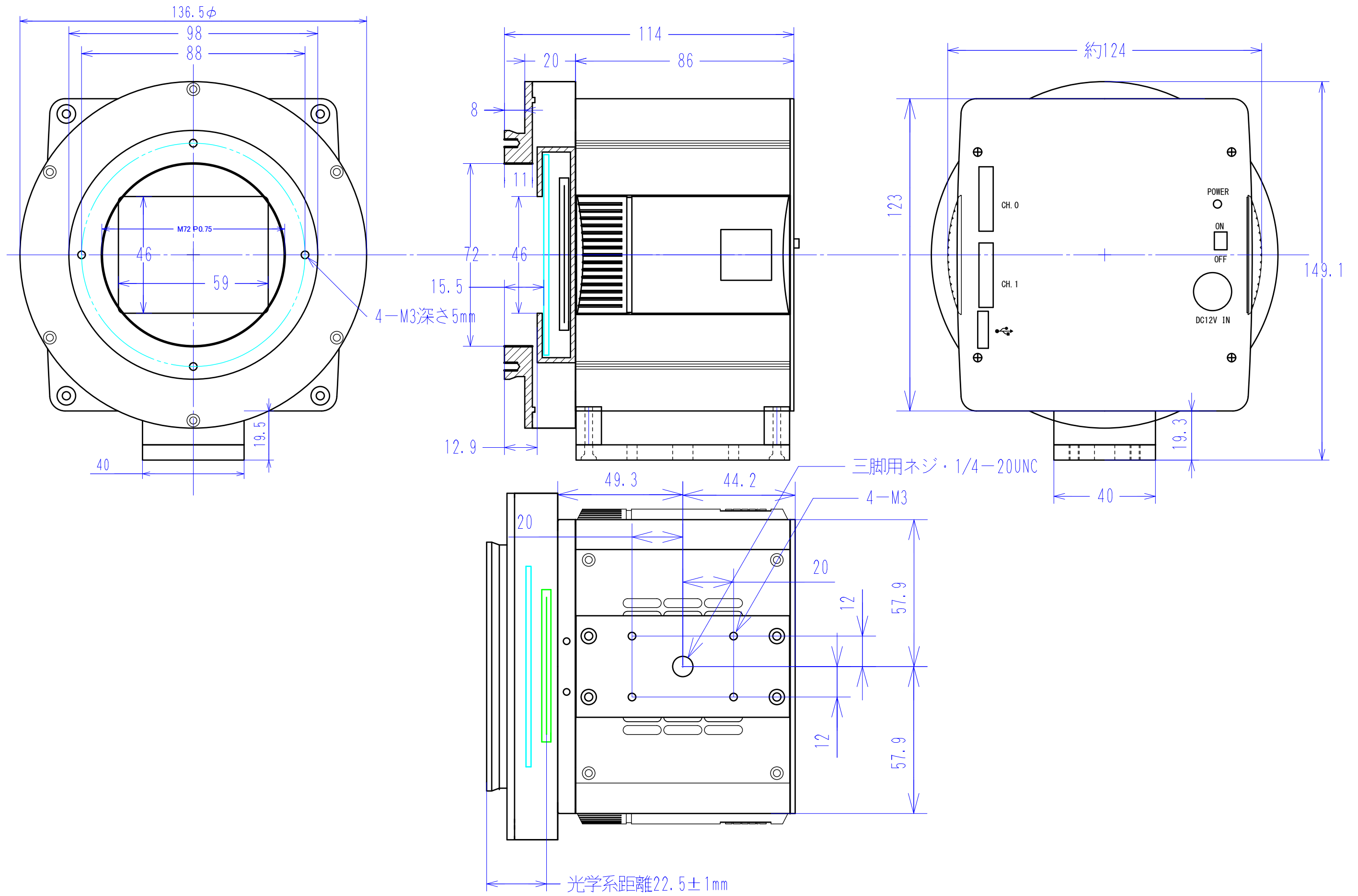
BH-66M 外観寸法図
