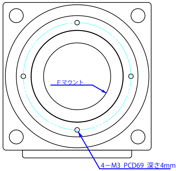
Fマウント正面
