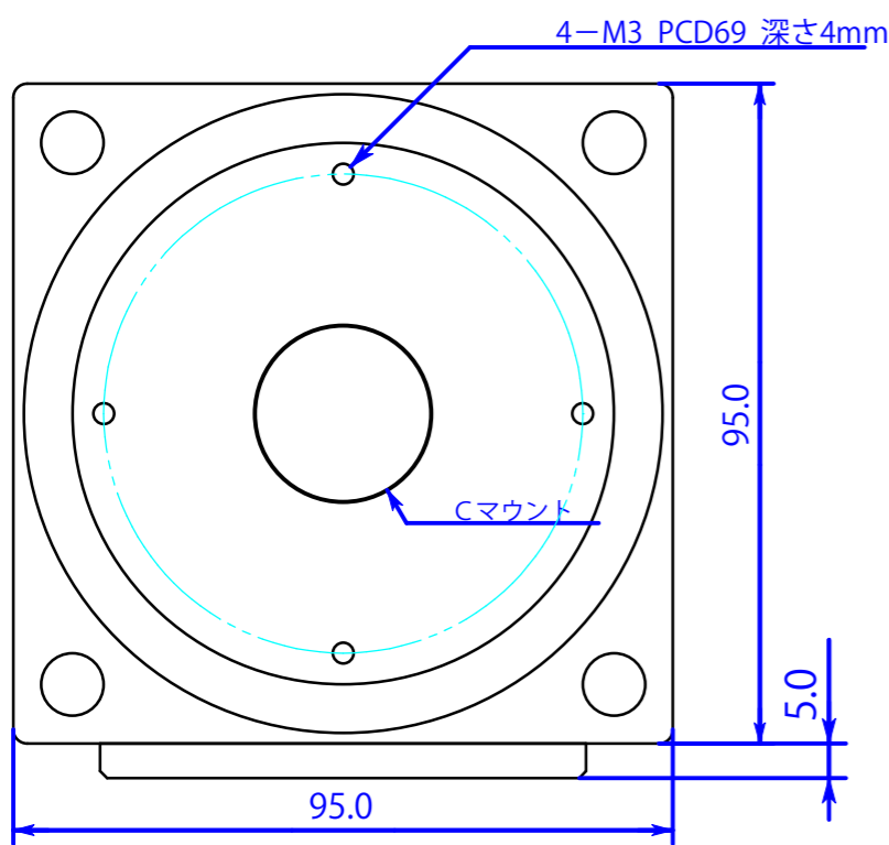
Cマウント正面
