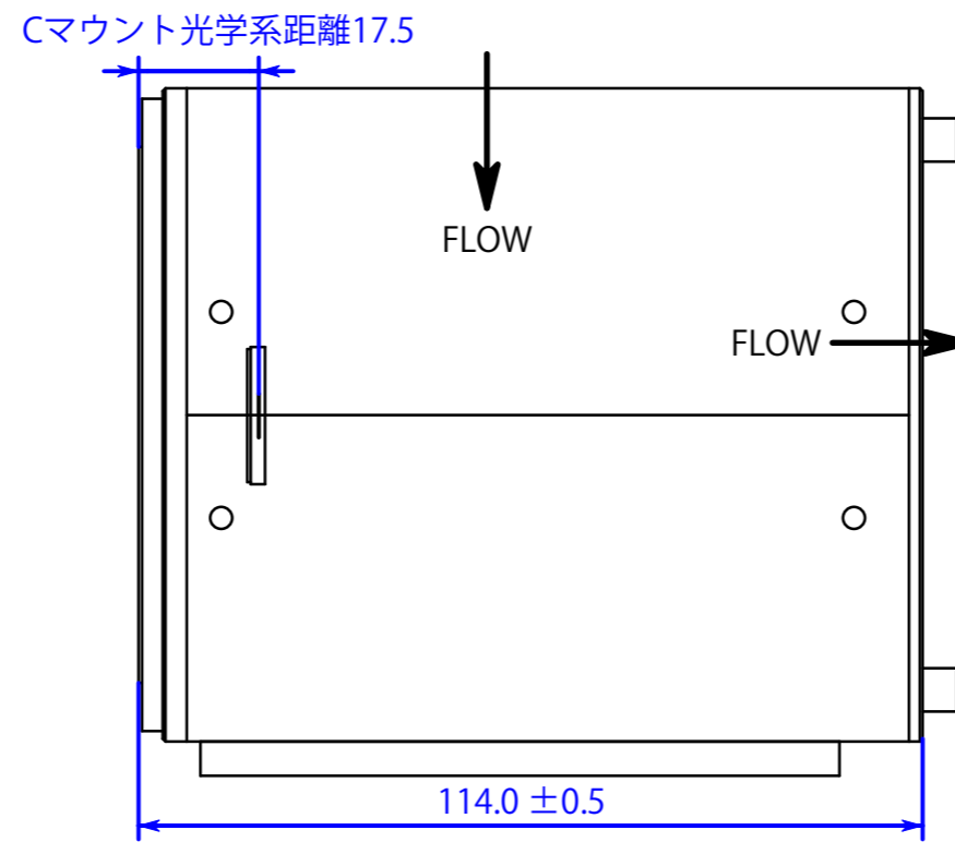
Cマウント側面
