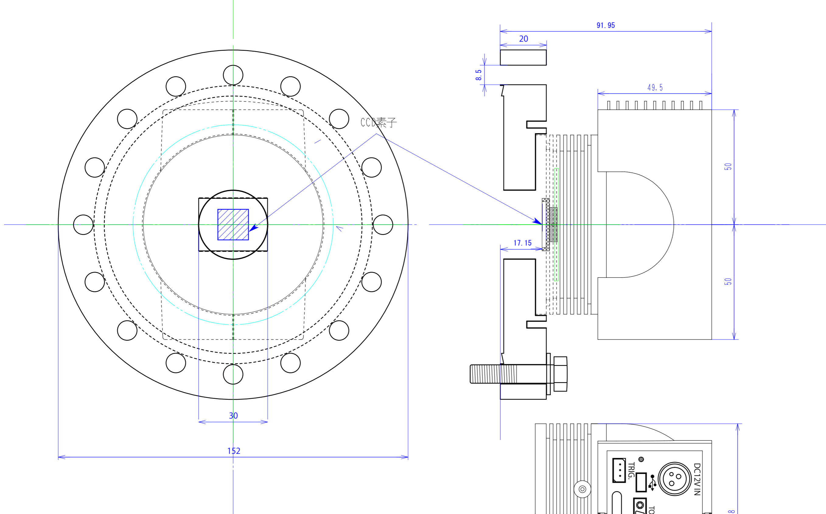
ICF152フランジ付き図面 フランジ側タップ無し
